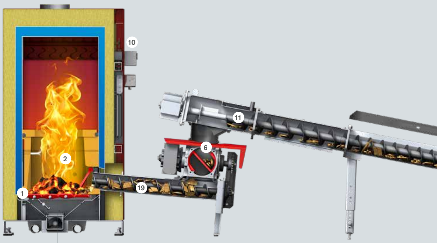
EcoHK 250 – 330, Vue avant
