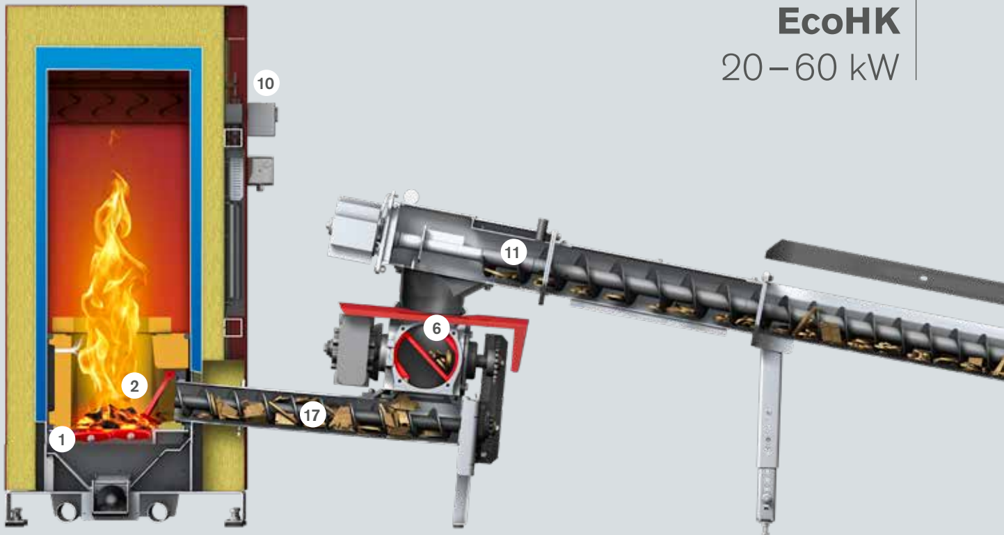
EcoHK 20–60, Vue avant
